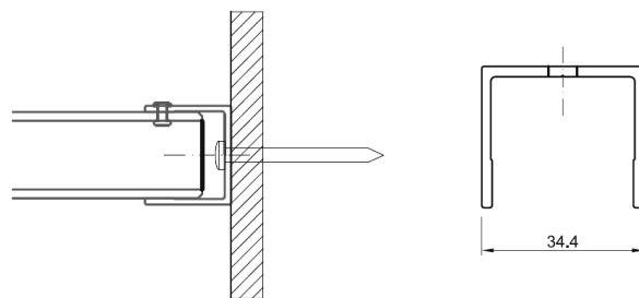
Profilé U
