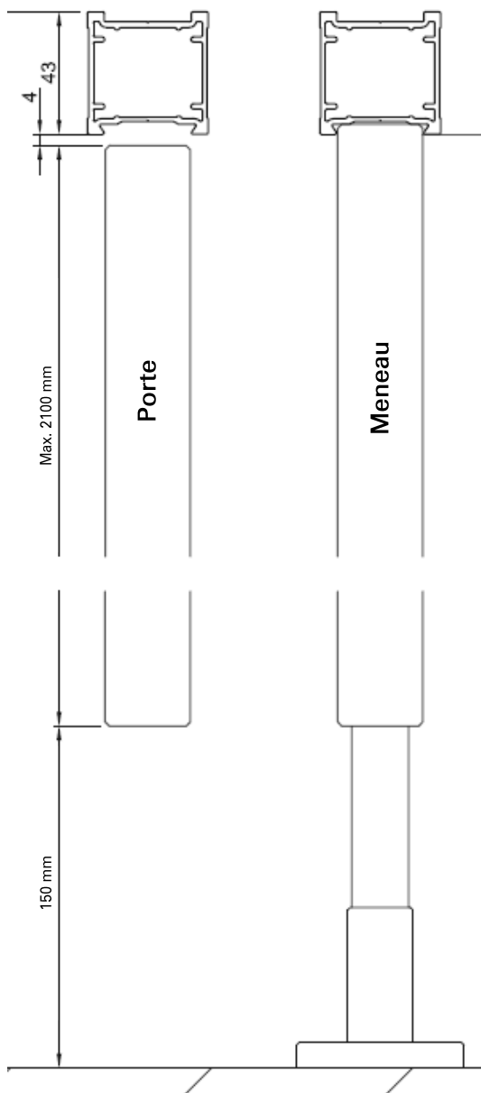
Coupe configuration standard
