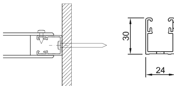
Profilé en joint-croix (option)
